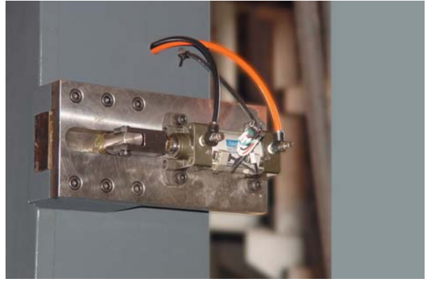
▲氣動式中座上極限安全鎖 Pneumatic slide TDC lock
