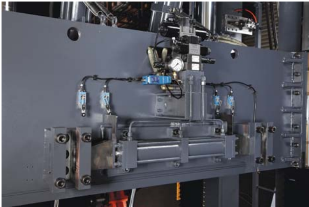
▲中座翻轉台盤油壓固定鎖 Slide table hydraulic lock
