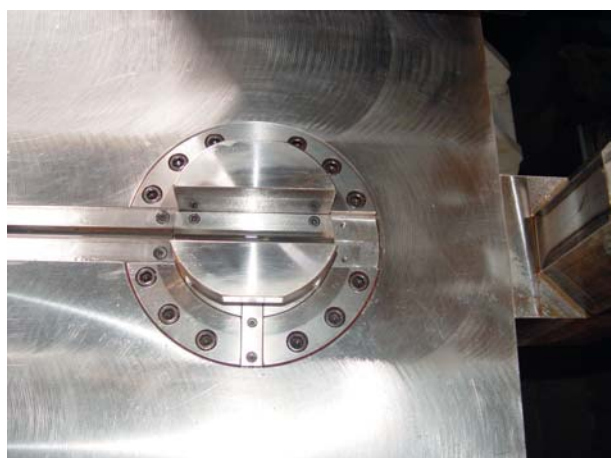
▲下工作台盤油壓定位鎖定系統 Bolster hydraulic positioning lock
